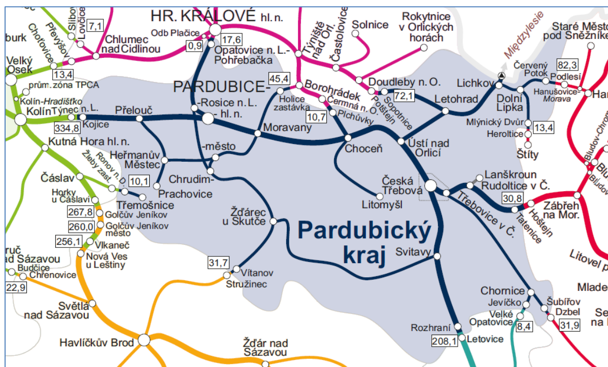
OBRAZEK 11 VÝŘEZ MAPY ŽELEZNIČNÍ SÍTĚ SE ZOBRAZENÍM ÚZEMÍ PARDUBICKÉHO KRAJE S INFORMACEMI O ČÍSLECH TRATÍ, POČTŮ TRATOVÝCH KOLEJÍ A NAPÁJECÍCH SOUSTAV, ZDROJ: SPRÁVA ŽELEZNIC
