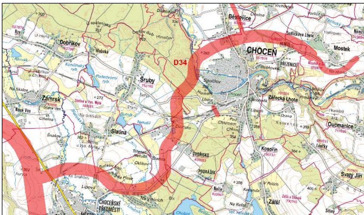
Obrázek 6: Vymezení koridoru D34 po vydání a nabytí účinnosti Aktualizace č. 3 ZÚR Pk (2020)
