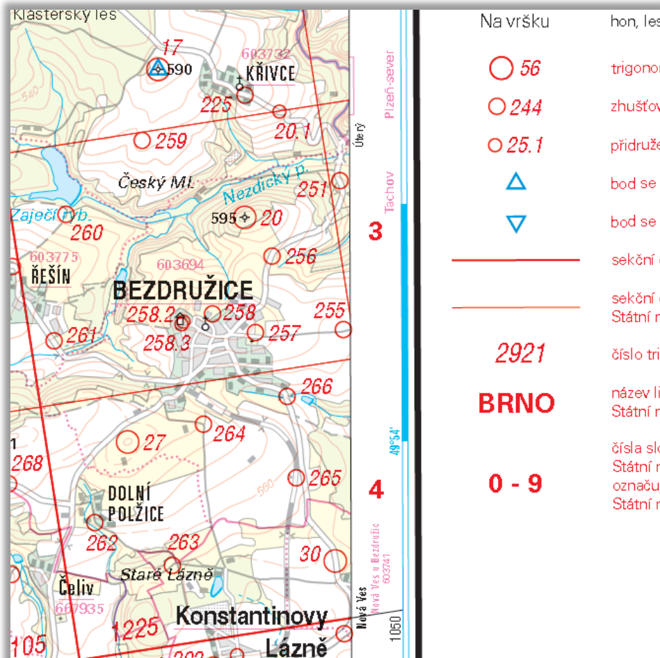
Přehled trigonometrických a zhušťovacích bodů 1 : 50 000 (z vlastních dat)
