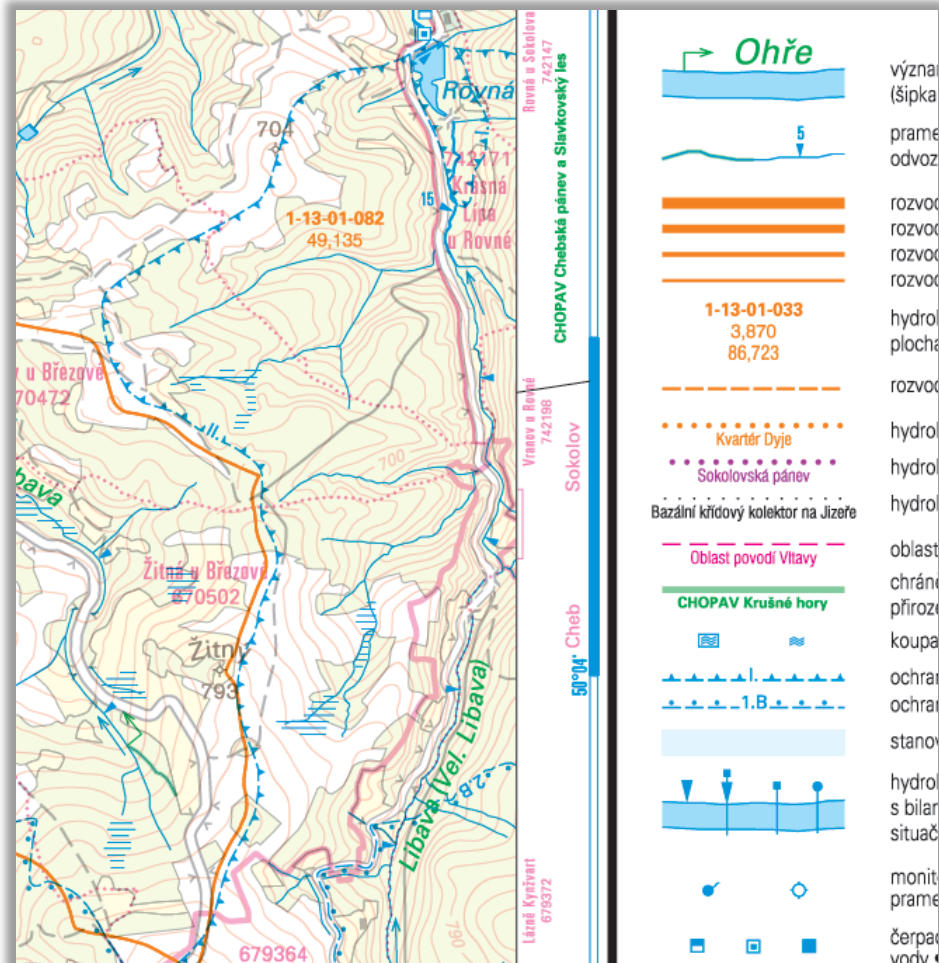
Základní vodohospodářská mapa 1 : 50 000 (z dat VÚV TGM)
