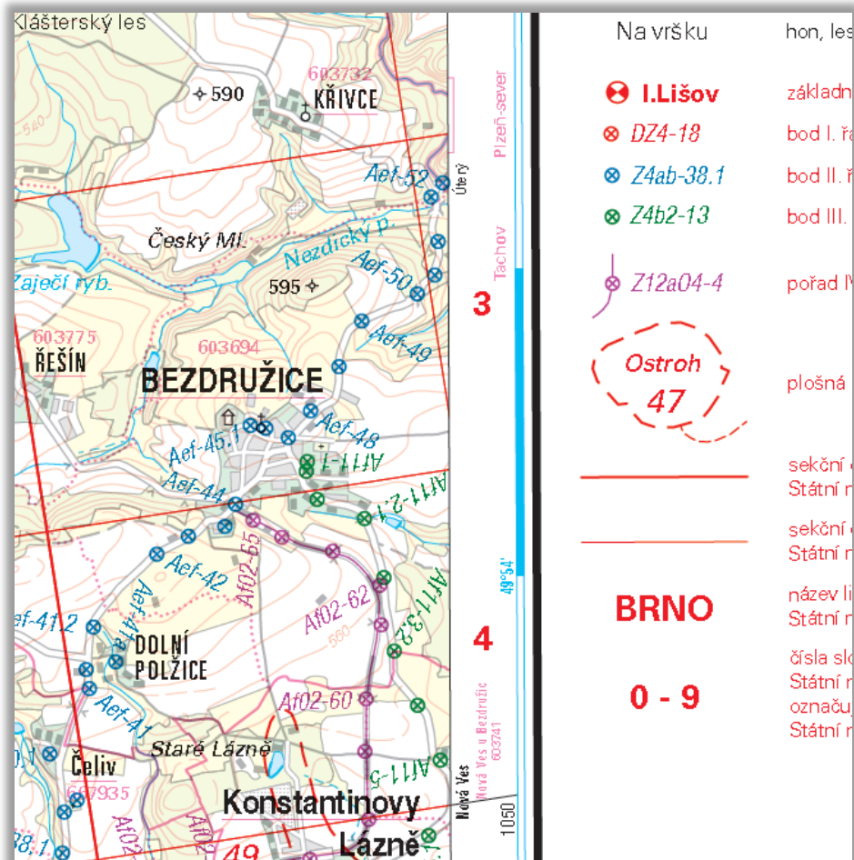
Přehled výškové (niveleční) sítě 1 : 50 000 (z vlastních dat)
