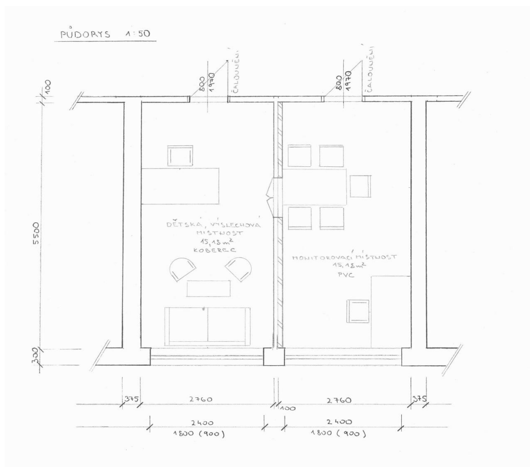
Obrázek č. 6: Půdorys speciálních vyšetřovacích místností ve Svitavách
